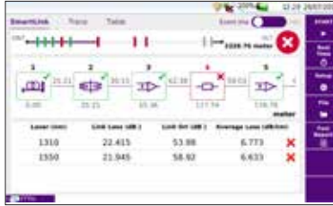
3 通过 SLM 自动显示，可轻松解读和分析
