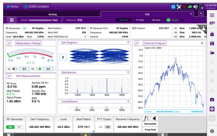
P25 测试界面和图表
