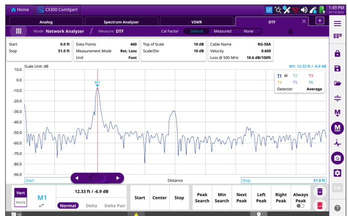
电缆和天线分析屏幕
