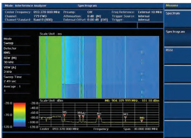
干扰分析测试 — 频谱图
