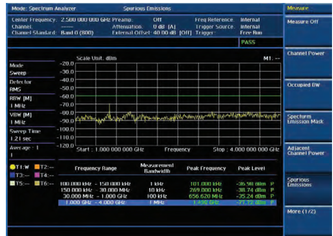
射频测试 — 杂散辐射
