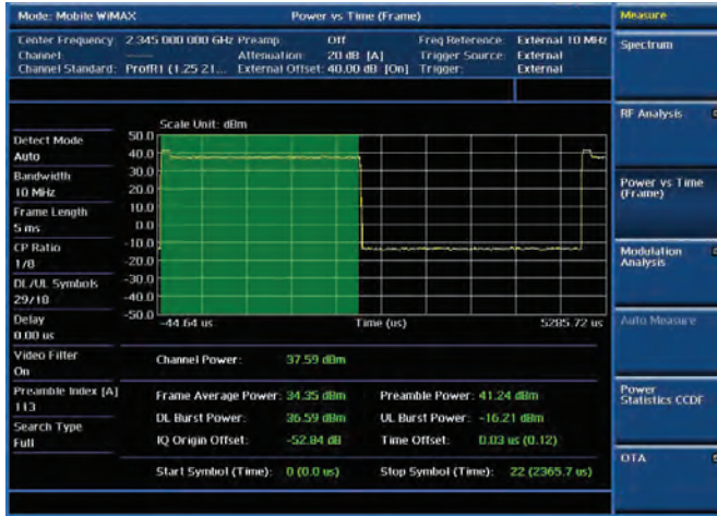
调制分析—功率与时间（帧）
