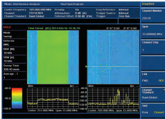
干扰分析测试 — 双频谱图
