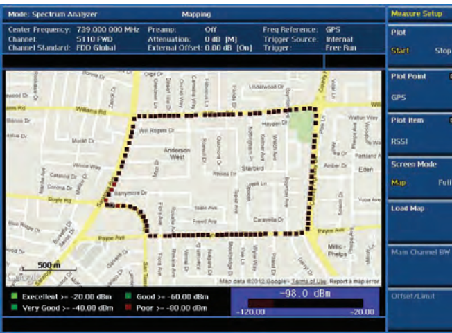
OTA 分析—线路图
