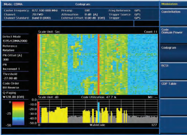
调制分析 — 码域功率瀑布图
