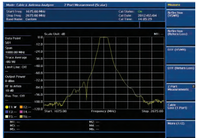
2 端口测量（标量）功能
