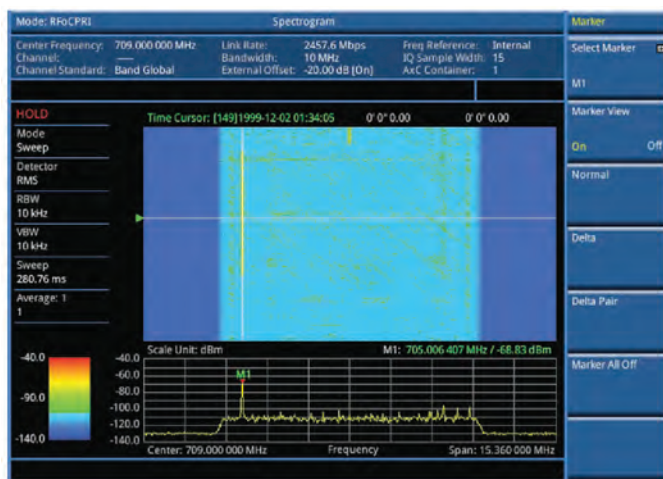
RFoCPRI - 频谱图
