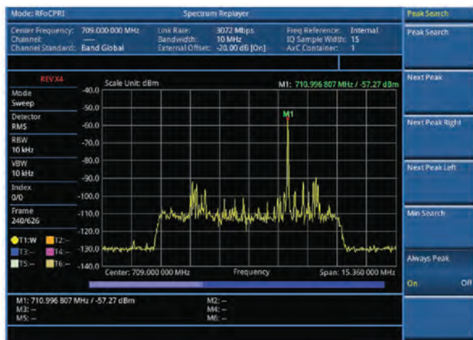
RFoCPRI - 频谱回放
