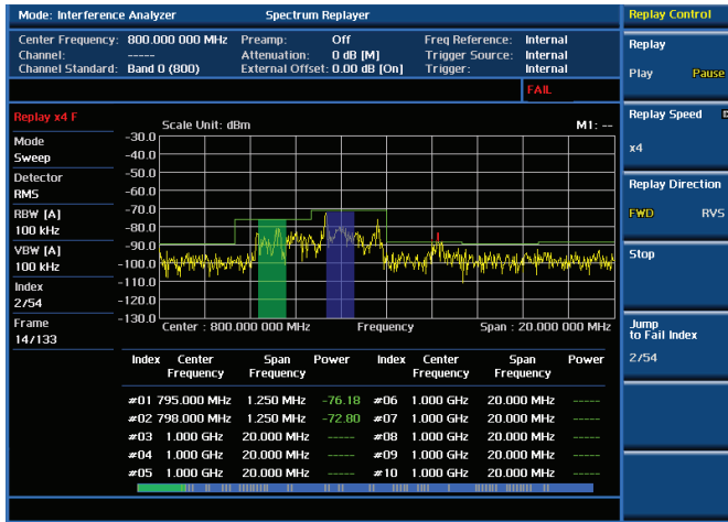
干扰分析测试 — 频谱回放
